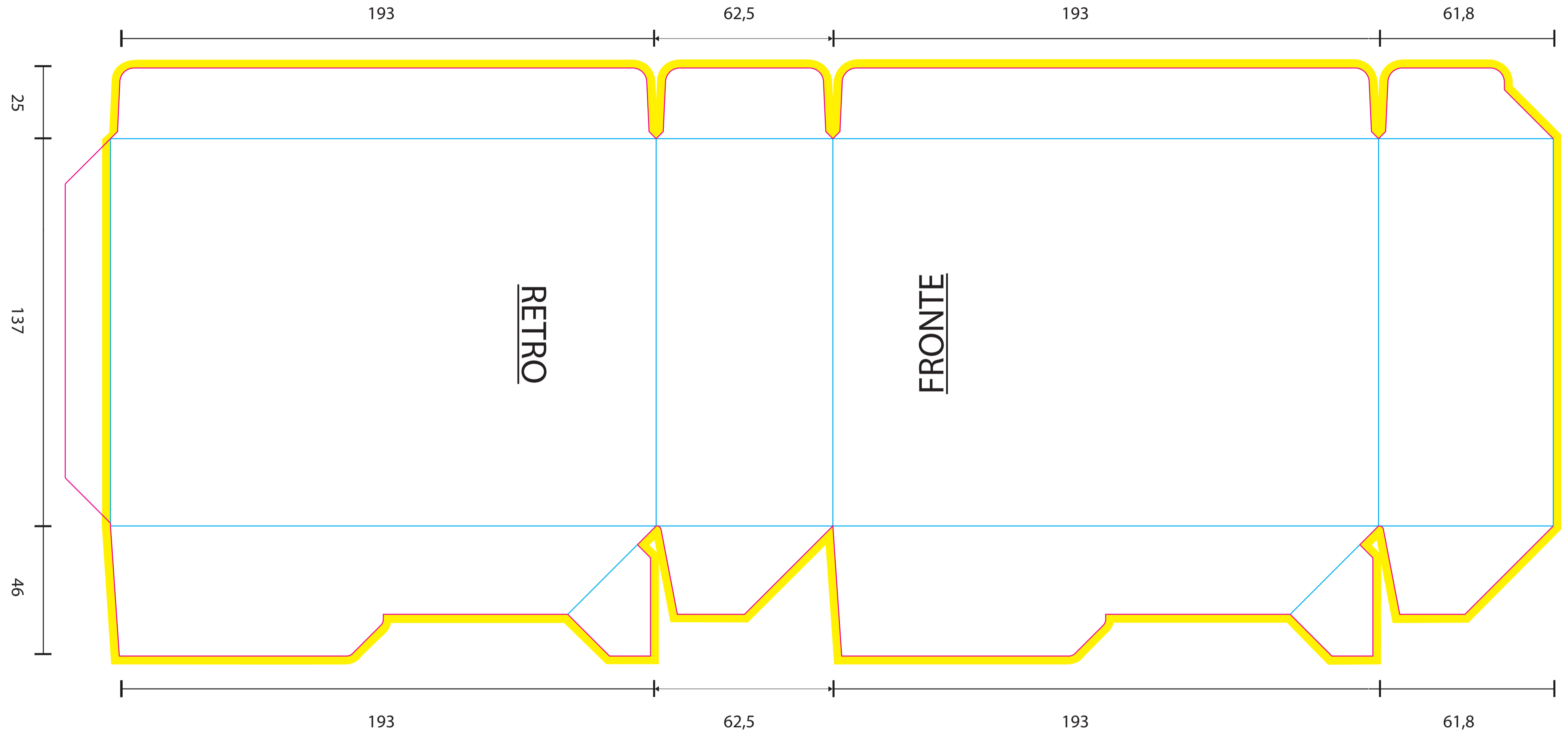
AR 0811 - CUSTODIA PER 4 BOX DVD con incollatura sul fondo
